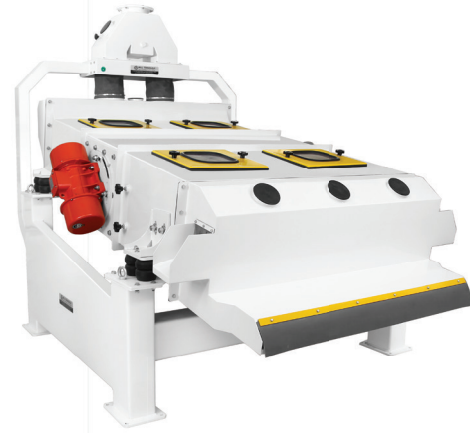
SEPARATEUR VIBRO SEPARATOR آلة الغربال الهزاز
