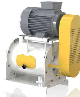
DETACHEUR A TAMBOUR DRUM DETACHER آلة المفقت الاسطوانى
