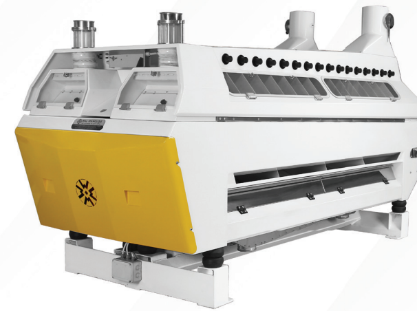
SASSEUR A SEMOULE SEMOLINA PURIFIER سيزند
