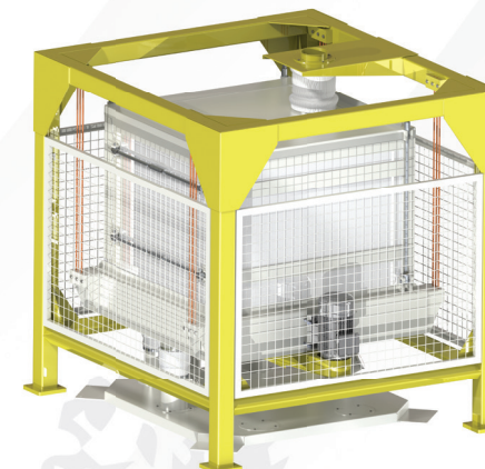
MONO CAISSE MONO SIFTER منخل كوتربول
